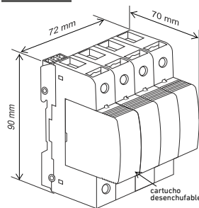
4 polos
