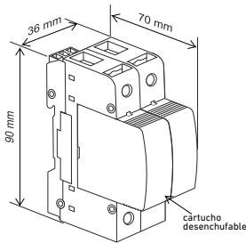
2 polos
